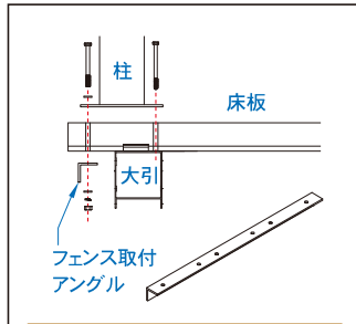
フェンス取付アングル
