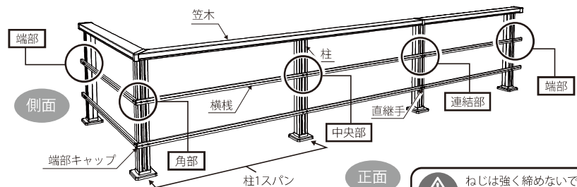
【AT-1型 横棧取付け方】
