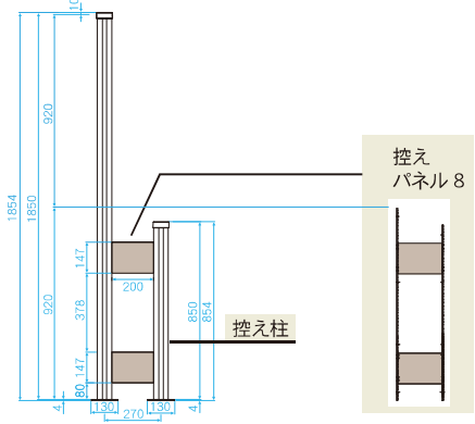
組立図
