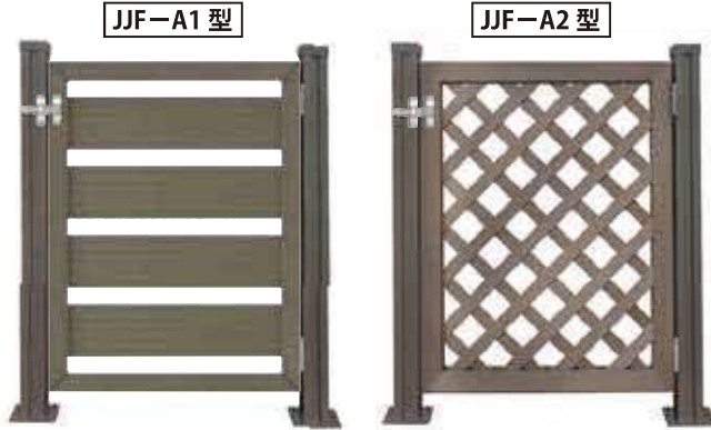
※H1000×W703( 柱芯心 800)
