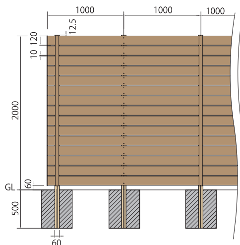
■基本寸法図
