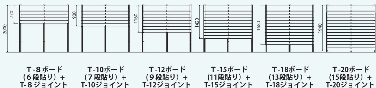
■ 組合せ例 (独立基礎施工用)
