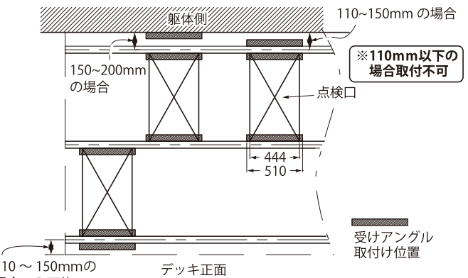
受えアングルの取付け
