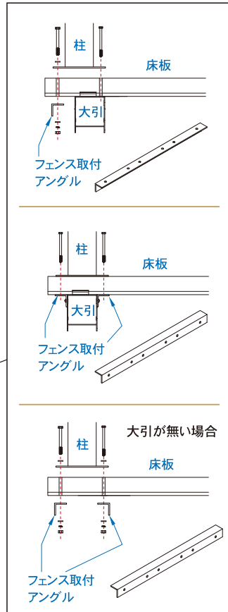
フェンス取付アングル
