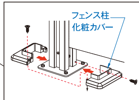
フェンス柱化粧カバー
