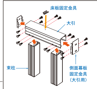
フレームB (独立)
