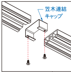
笠木連結キャップ
